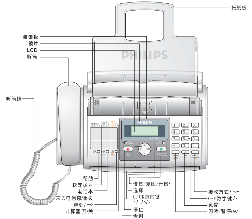
1.4 控制面板:
